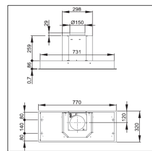
Dimension 770
